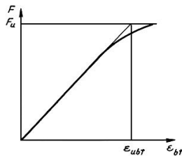
F - нагрузка; F_u - разрушающая нагрузка; \epsilon_{dt} - деформация растянутой поверхности образца; \epsilon_{ubt} - предельная относительная деформация растяжения
